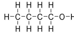
Butanol
